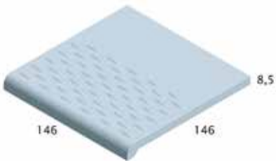
ST Askelmalaatta 66 + väri + ST
