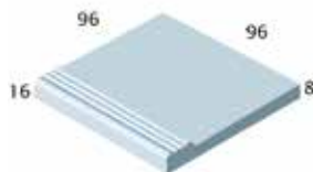
PES Allasreunalaatta, sileä 44 + väri + PES
